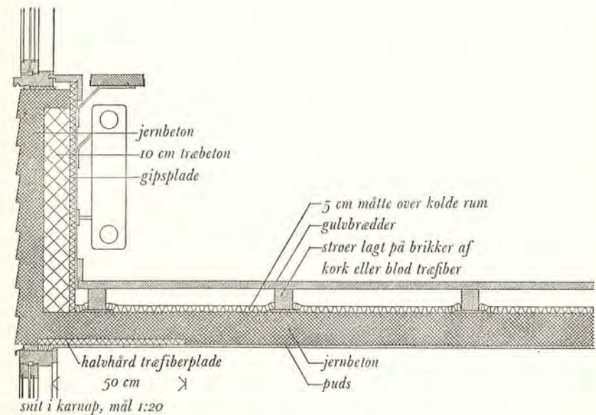
Fig. 21. Isolering af radiatorbrystning ved karnapaltan.
