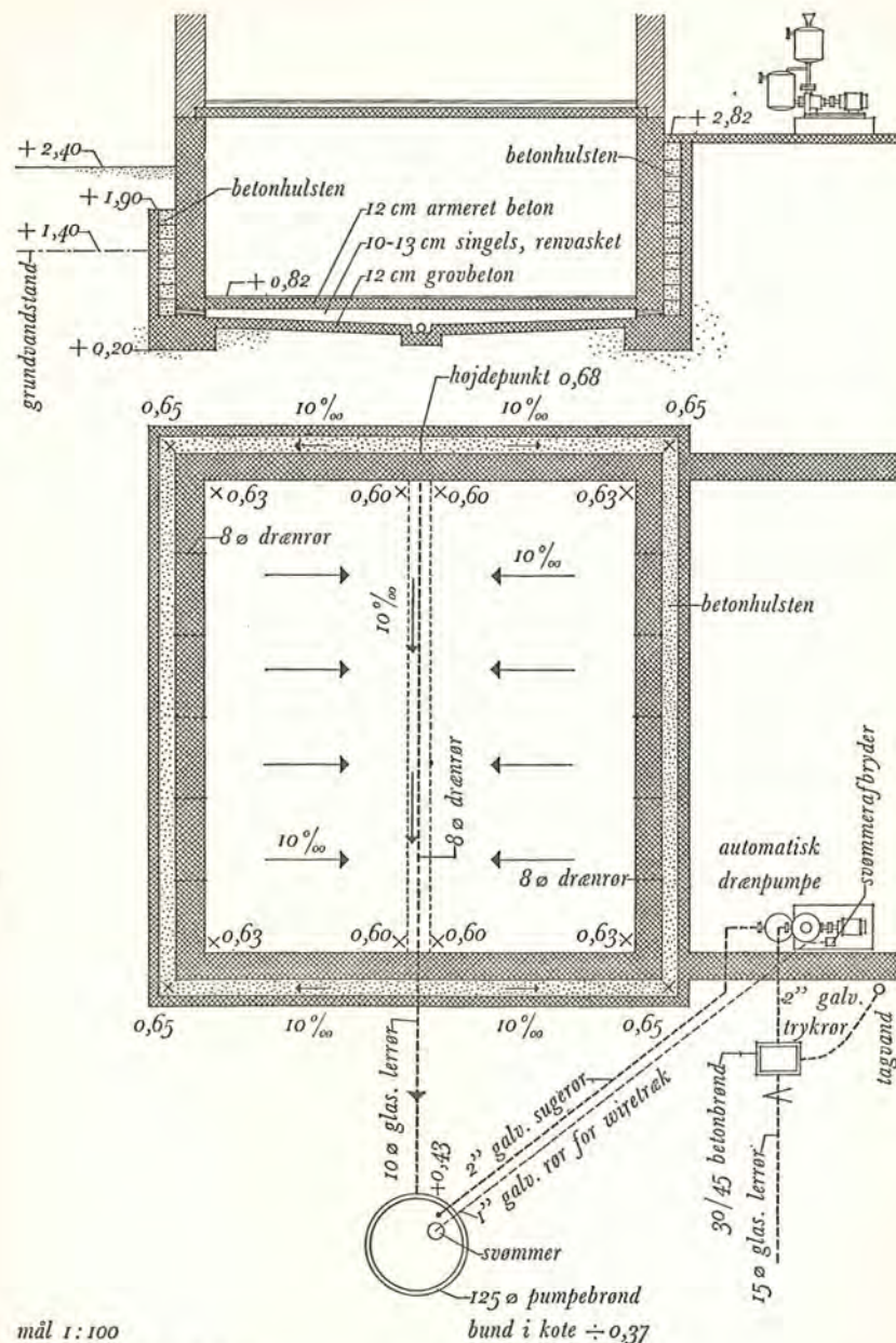
Fig. 5. Indskudsdræn.
