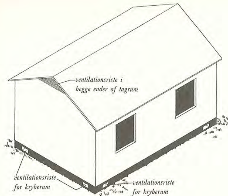
Fig. 22. Ventilation af tagrum under tæt tag.
