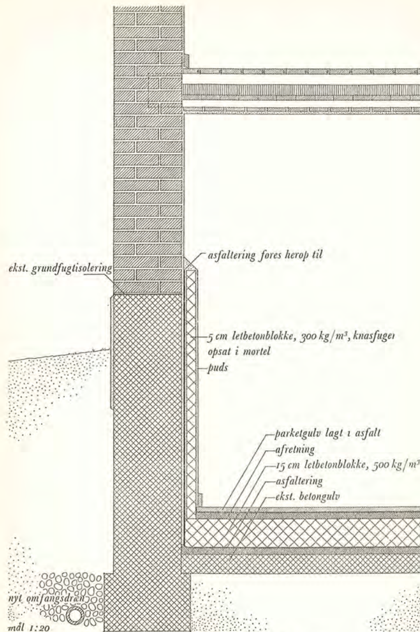
Fig. 4. Indretning af eksisterende kælder til arbejdsrum.
