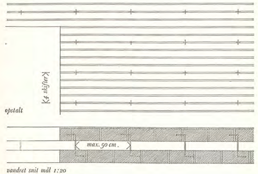
Fig. 14. Bindere til hule mure.
