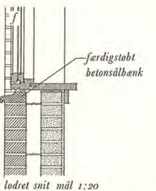
Fig. 13. Vinduer i hule mure.
