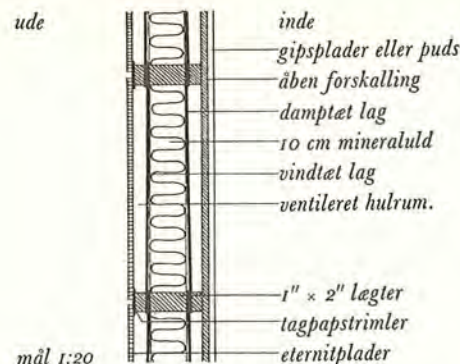
Fig. 20. Træskeletvæg (vandret snit).
