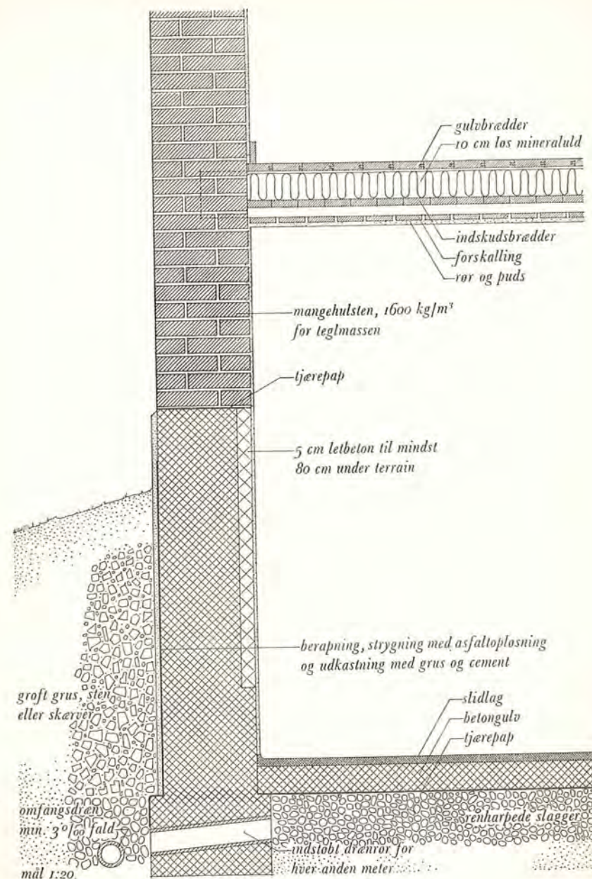
Fig. 2. Fugtisolering af kælderydervæg.
