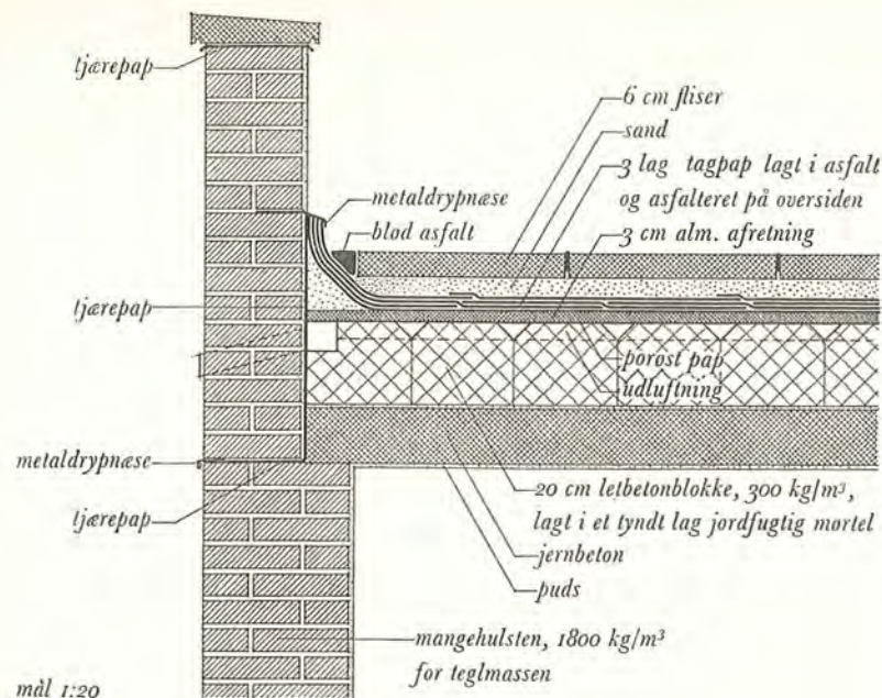
Fig. 24. Massivt tag med murkrone ved fuld mur af teglsten.
