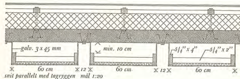
Fig. 31. Tag over lokale med fugtig varm luft.
