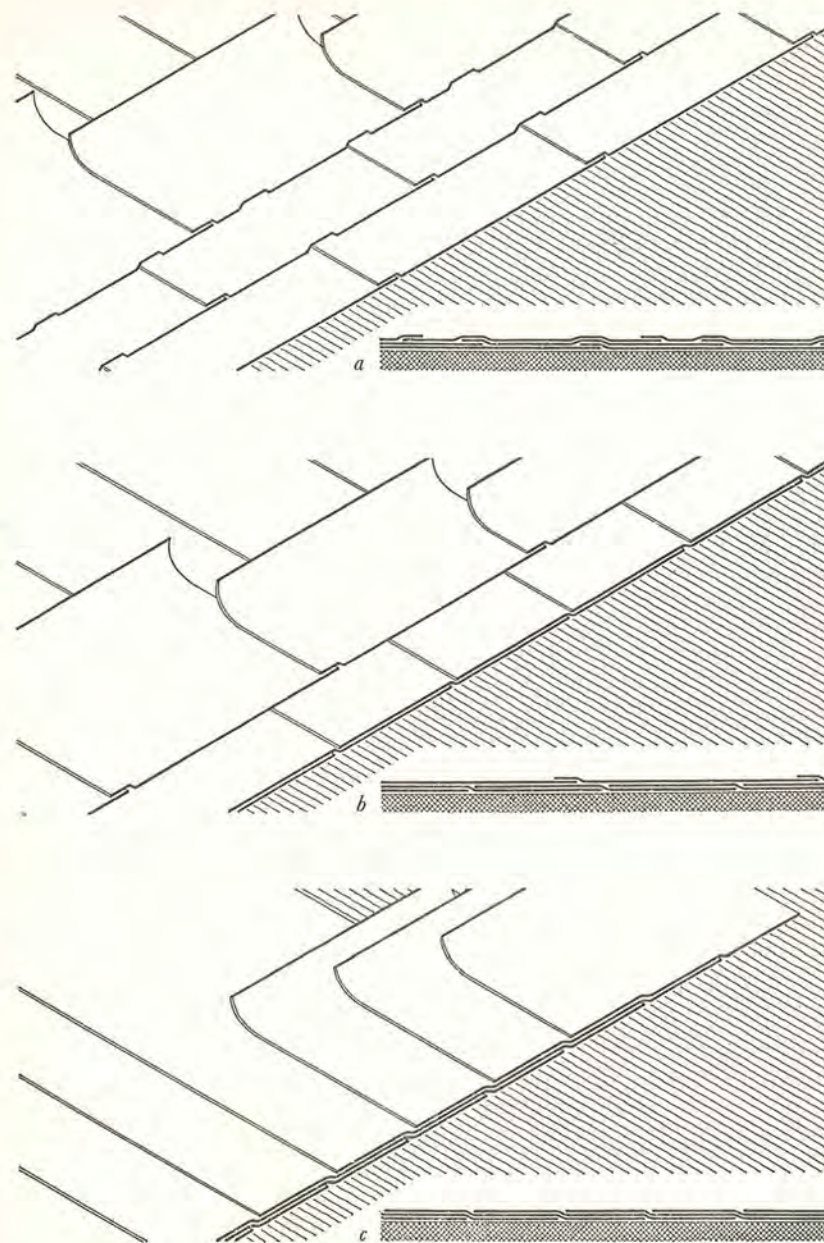
Fig. 29. Tækning af massive betontage.
