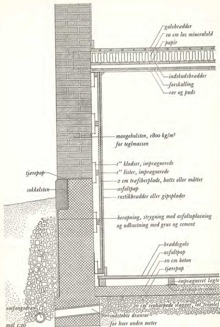
Fig. 3. Indretning af ny kælder til arbejdsrum.
